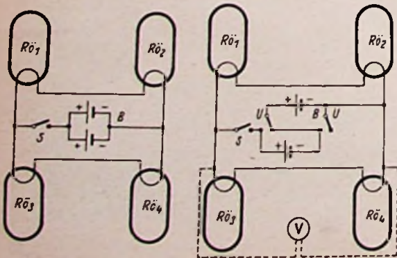
Rechts: Bild 2. Zweipoliger Umschalter zur Serien- oder Parallelschaltung der beiden Taschenlampenbatterien B. Heizstromentnahme bei Serienschaltung = 120 mA (U = zweipoliger Umschalter, V = Voltmeter zur genauen Spannungskontrolle).
