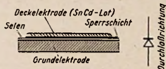
Bild 1. Aufbau eines Selen-Trockengleichrichters
