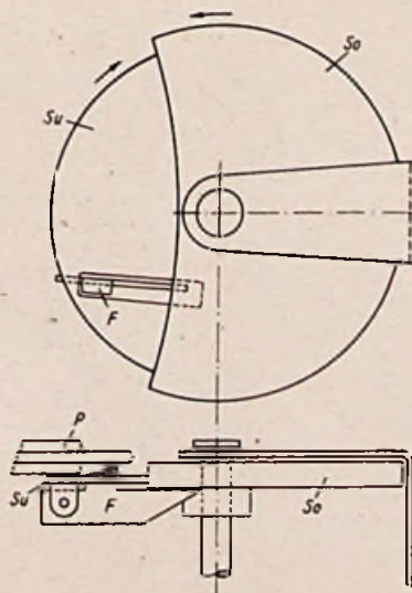
Bild 6. Dual-Fühlhebelmechanismus
